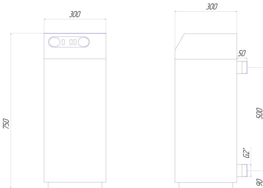
Мал. Електрокотел WPG 9-30 кВт 380в
